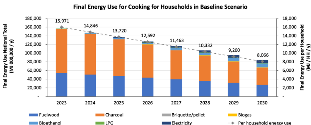
Figure 29. Consommation d'énergie finale pour la cuisson des aliments par les ménages dans le scénario de base
