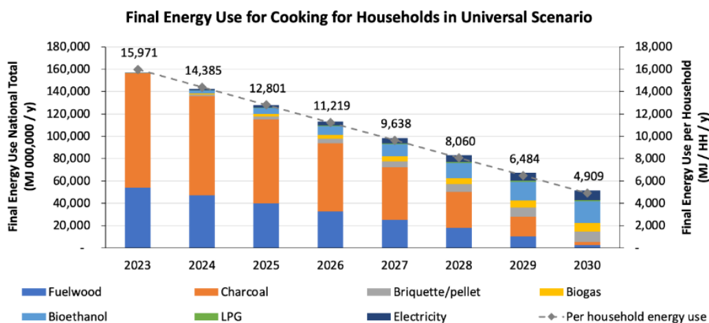
Figure 31. Consommation d'énergie finale pour la cuisson des aliments dans les ménages selon le scénario universel
