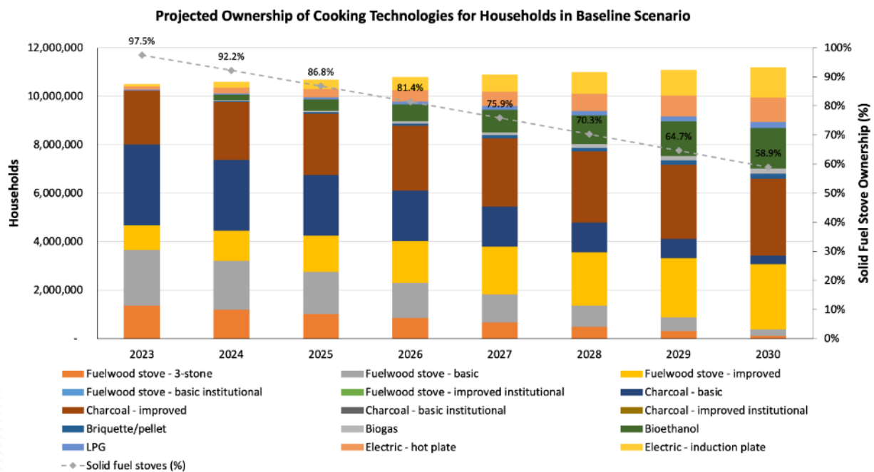
Figure 20. Projection de la possession de technologies de cuisson pour les ménages dans le scénario de base
