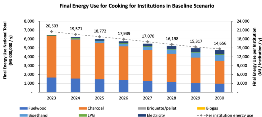
Figure 30. Consommation d'énergie finale pour la cuisson dans les institutions dans le scénario de base
