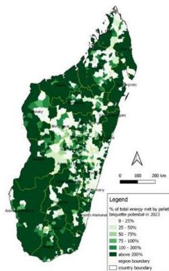
Figure 15. Potentiel des besoins totaux en énergie de cuisson pouvant être satisfaits par le potentiel de production de granulés/briquettes de biomasse dans chaque commune en 2023.
