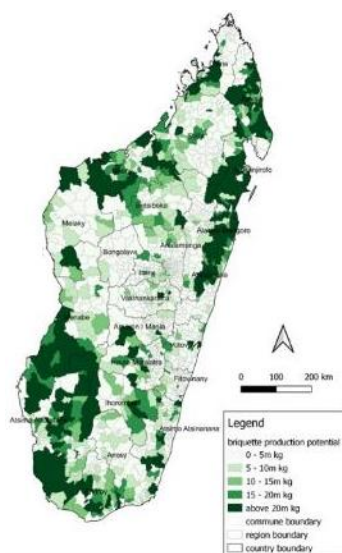
Figure 14. Potentiel de production de granulés/briquettes de biomasse.
