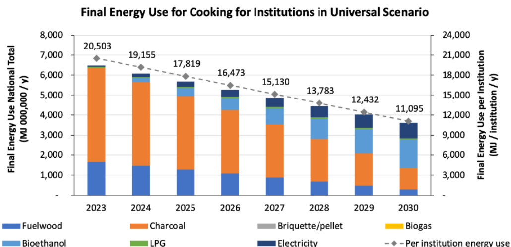
Figure 32. Consommation d'énergie finale pour la cuisson dans les institutions selon le scénario universel
