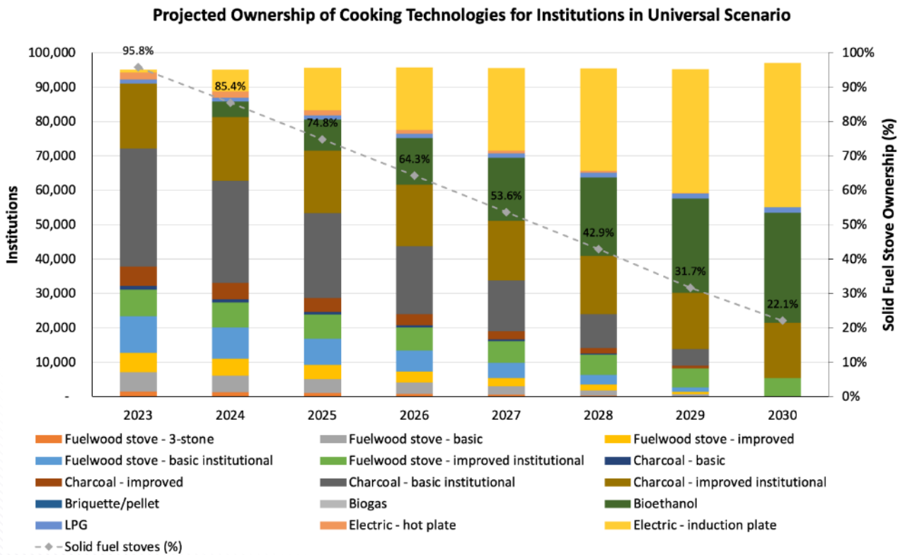
Figure 26. Projection de la possession de technologies de cuisson pour les institutions dans le scénario universel
