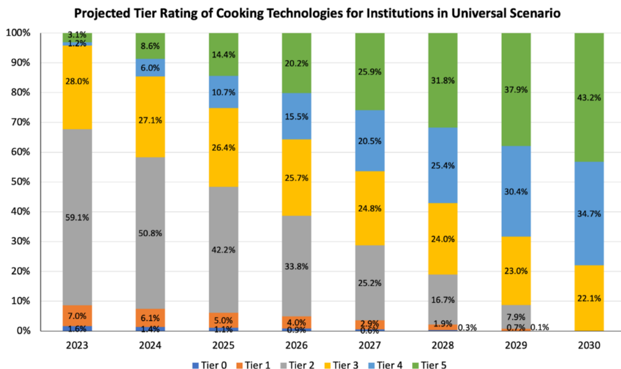
Figure 27. Classement par niveau des technologies de cuisson pour les institutions dans le scénario universel
