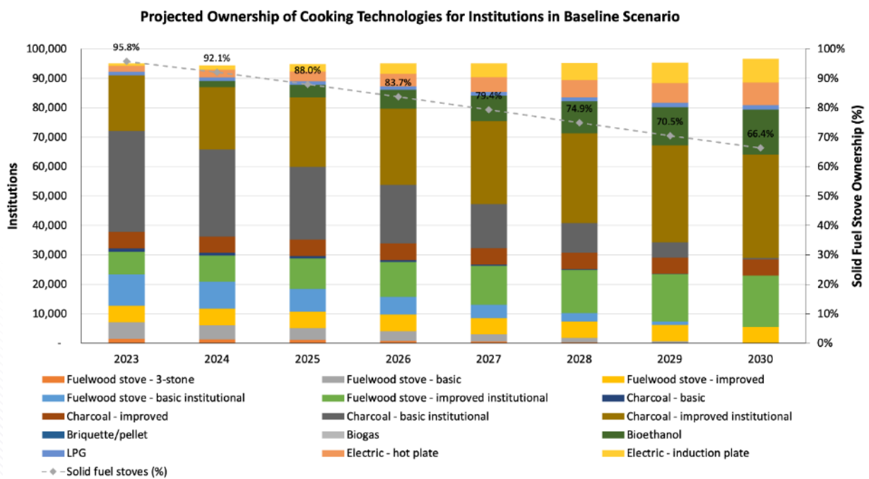
Figure 24. Propriété projetée des technologies de cuisson pour les institutions dans le scénario de base
