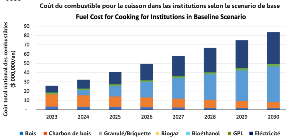
Figure 36. Coût total national des combustibles pour la cuisson dans les institutions selon le scénario de base
